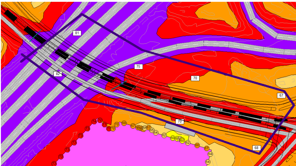
Kuva 7. Raitiotie- ja tieliikenteen aiheuttamat päiväaikaiset keskiäänitasot (LAeq 7-22) asemakaavan eteläisessä osassa ennustetilanteen liikennemäärillä (v. 2040).
