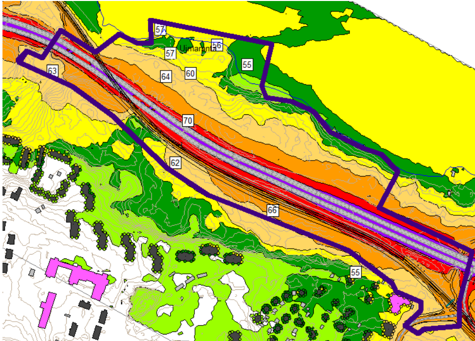
Kuva 5. Raitiotie- ja tieliikenteen aiheuttamat päiväaikaiset keskiäänitasot (LAeq 7-22) ennustetilanteen liikennemäärillä (v. 2040).
