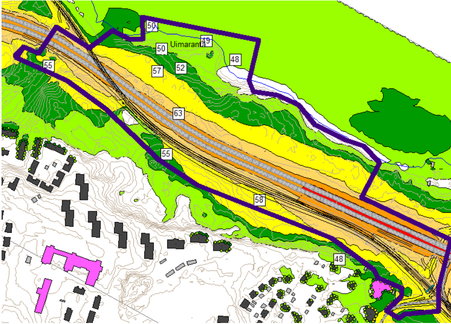
Kuva 6. Raitiotie- ja tieliikenteen aiheuttamat yöaikaiset keskiäänitasot (LAeq 22-7) ennusteliikenteen liikennemäärillä (v.2040).
