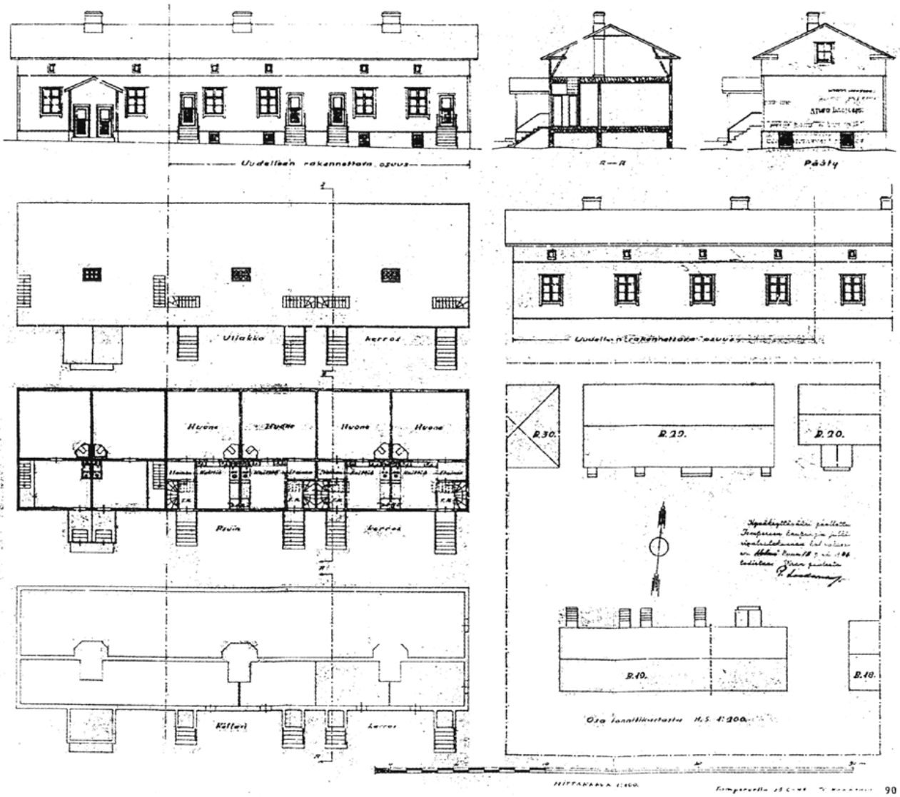
Kuvassa Masuuninmäen asuinrakennuksen B 19 piirustukset.
