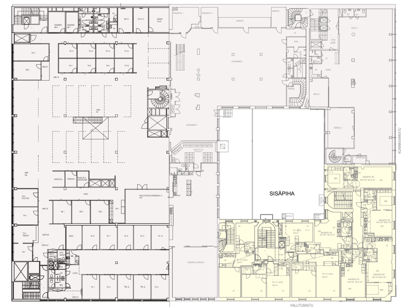
3.-KERROS
