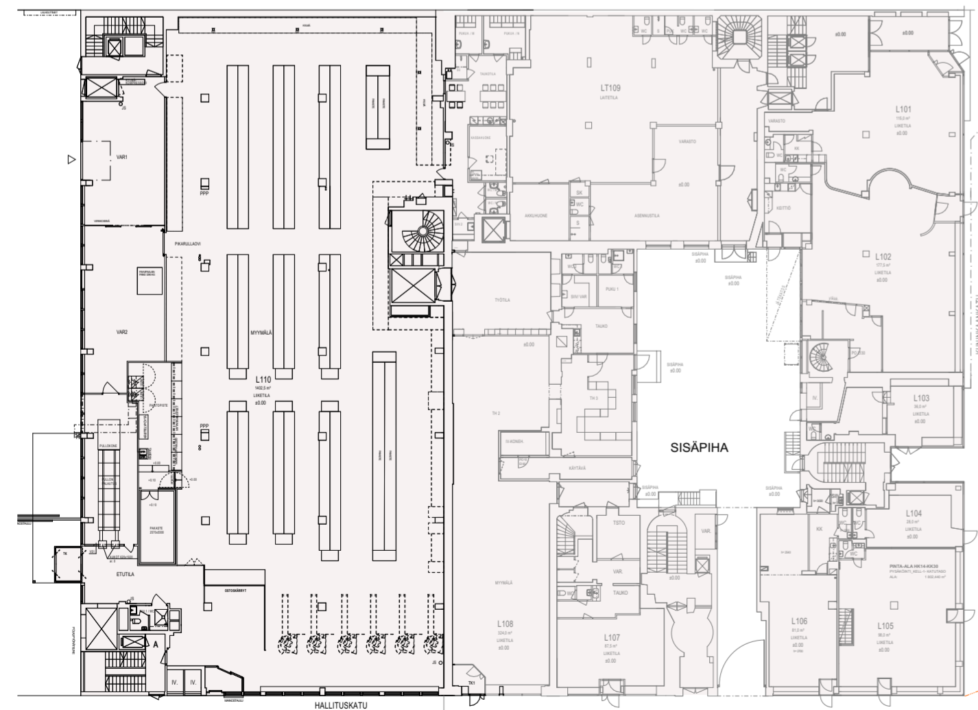
1.-KERROS
