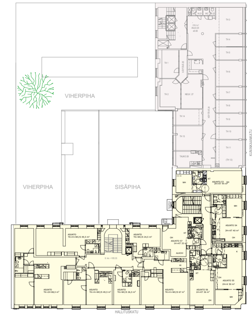
6.-KERROS
