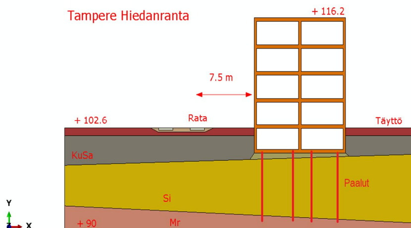
Kuva 2. Laskentapoikkileikkaus mallinnuksessa.
