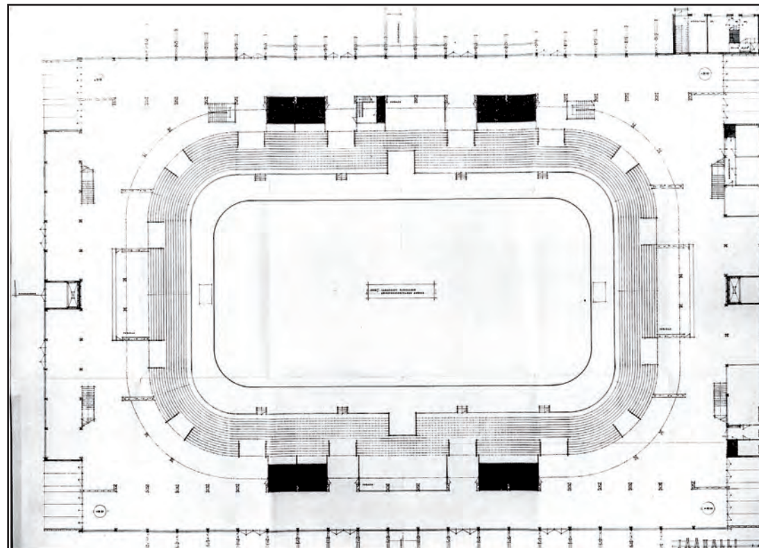
Kenttätason ja sisäänkäyntitason pohjapiirustukset vuodelta 1964.
