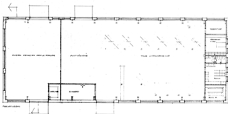
Puutyöpajan alkuperäinen pohjapiirros
