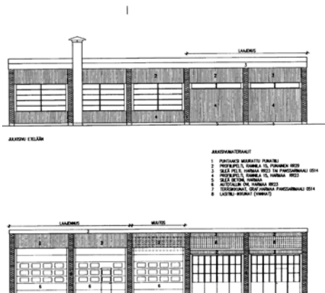
Autosuojarakennuksen muutospiirrokselta vuodelta 2006
