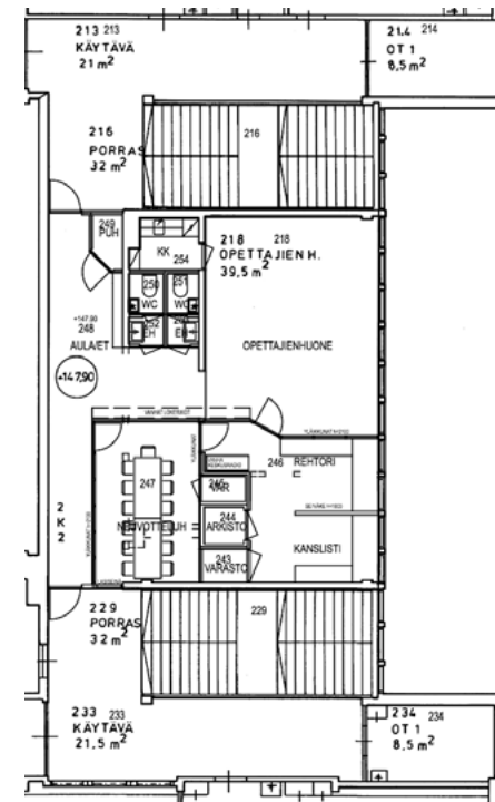
Pohjapiirustusote, 2.kerros. Hallintotilojen muutos, uudet erityisopetustilat käytävien päissä.
