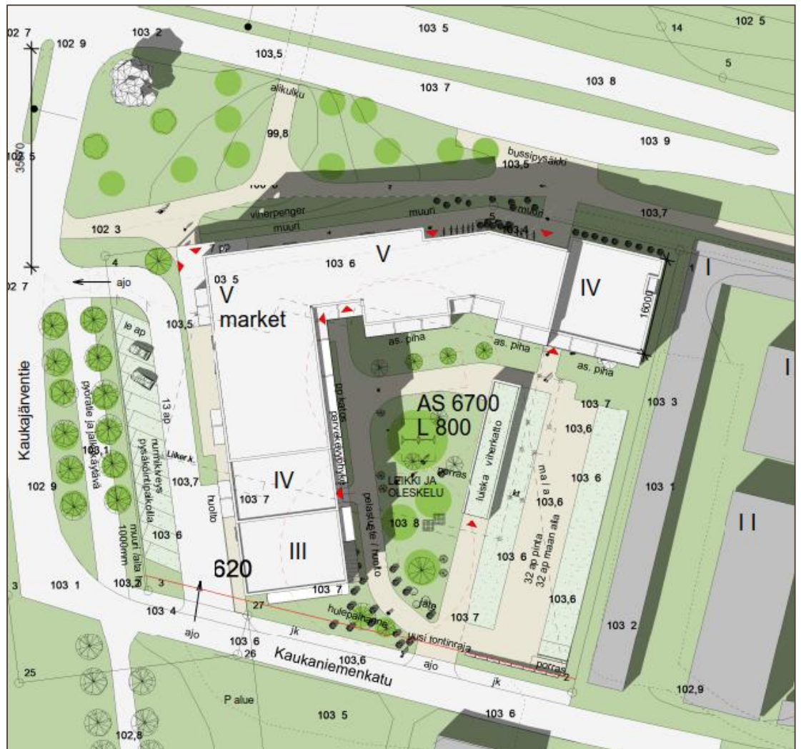
Kuva 1. Kohteen asemapiirros.
