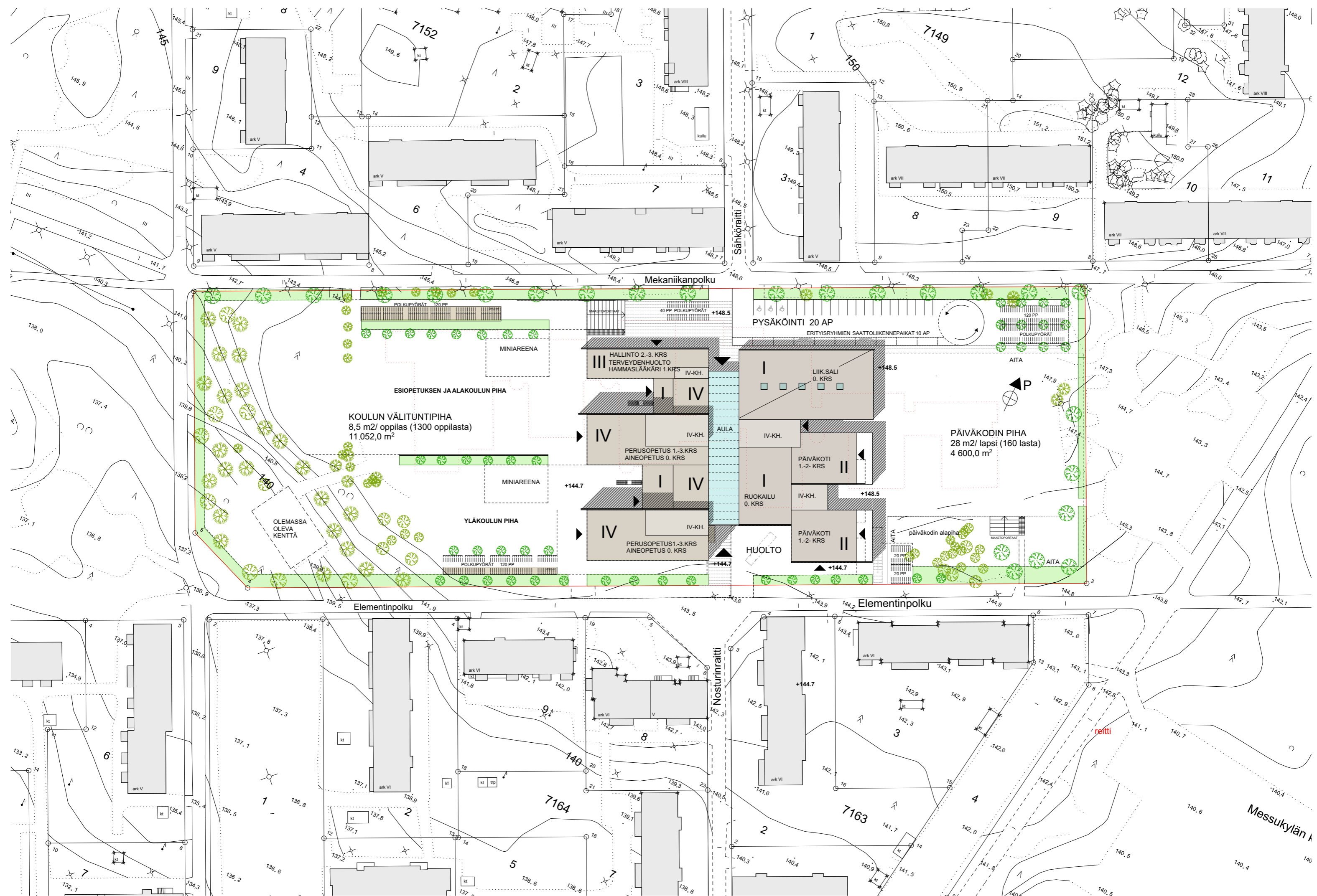
ETELÄ-HERVANNAN KOULU JA PÄIVÄKOTI, UUDISRAKENNUS, TONTINKÄYTTÖLUONNOS 1:1000, ARKITEHTITOIMISTO TILATAKOMO 16.10.2018
