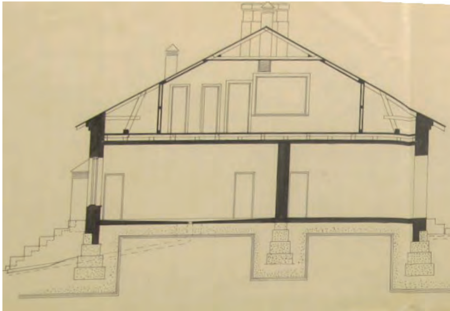
Leikkaus.
