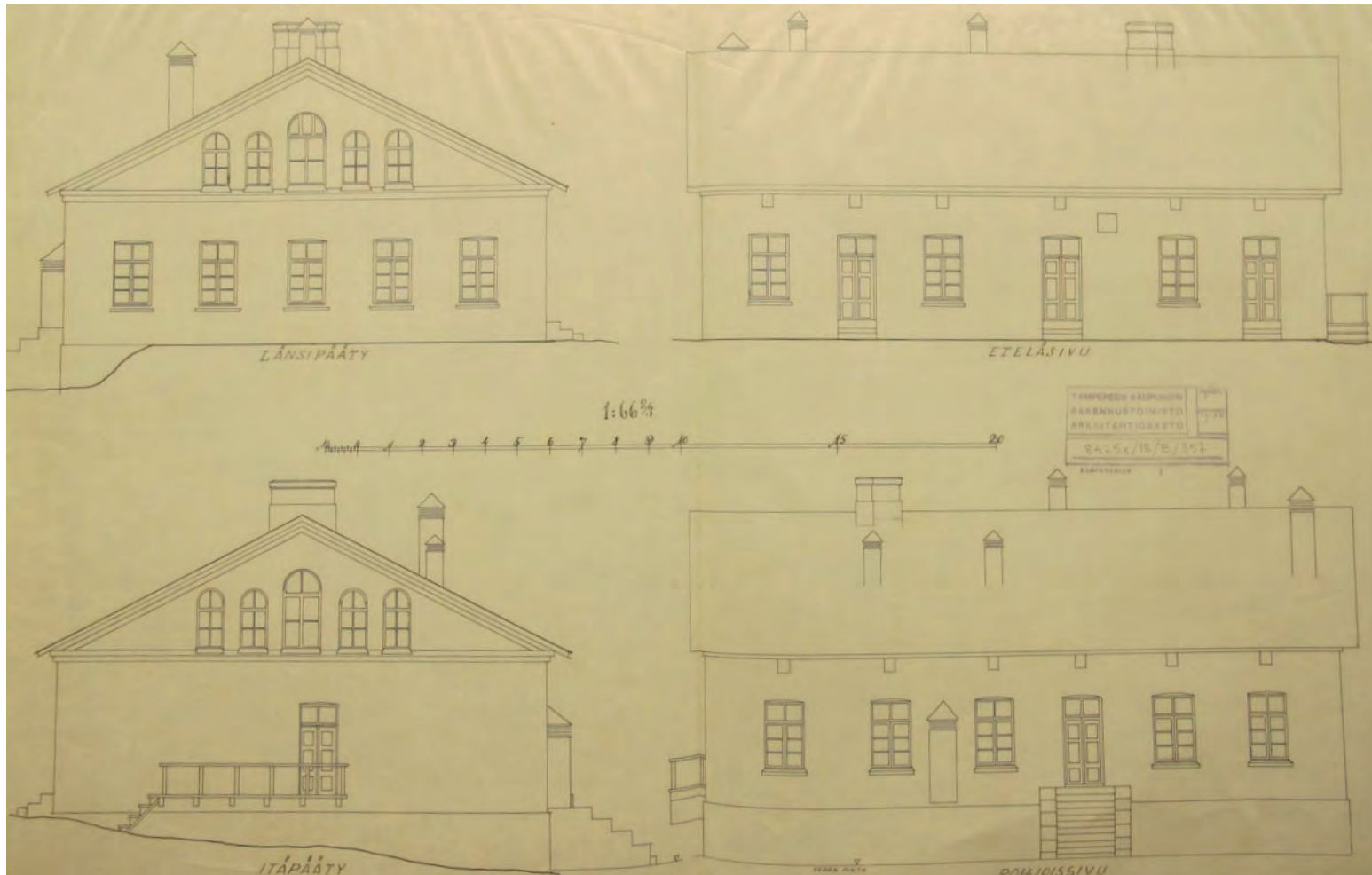
Alkuperäiset julkisivut.
