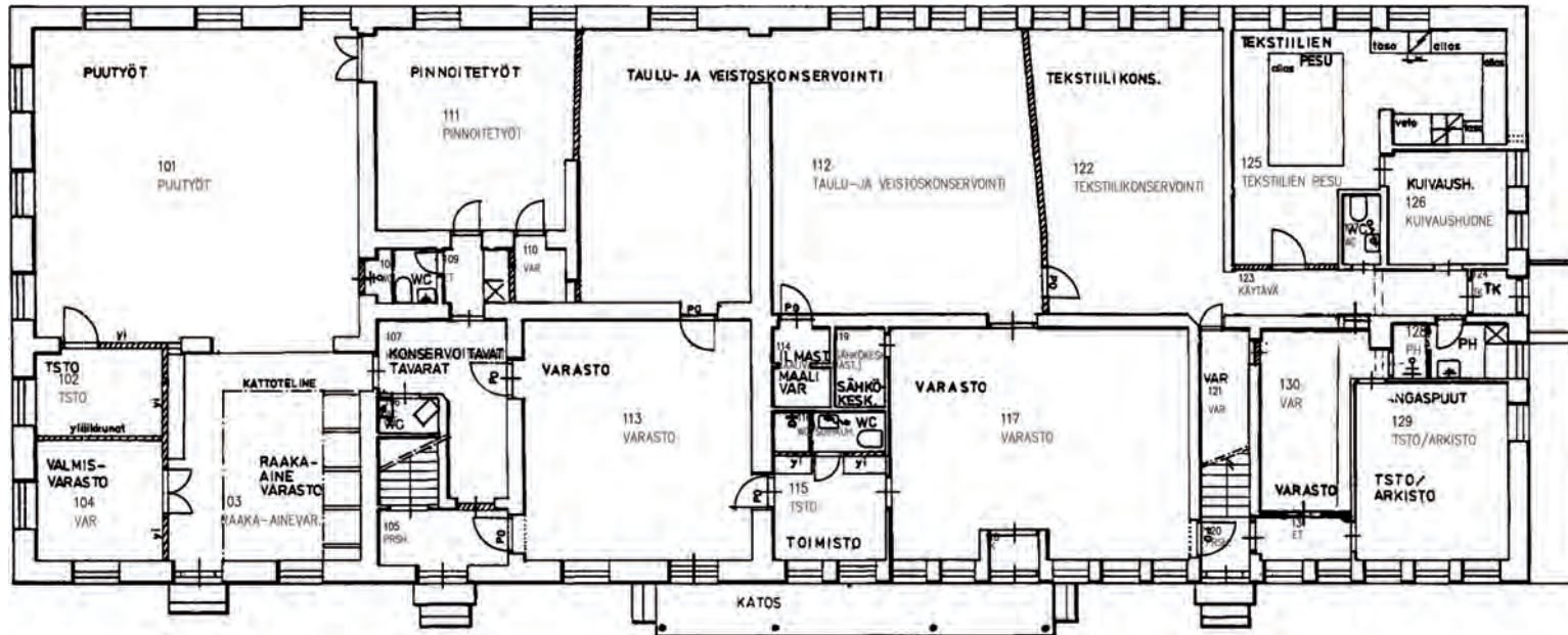
Pääkerros
