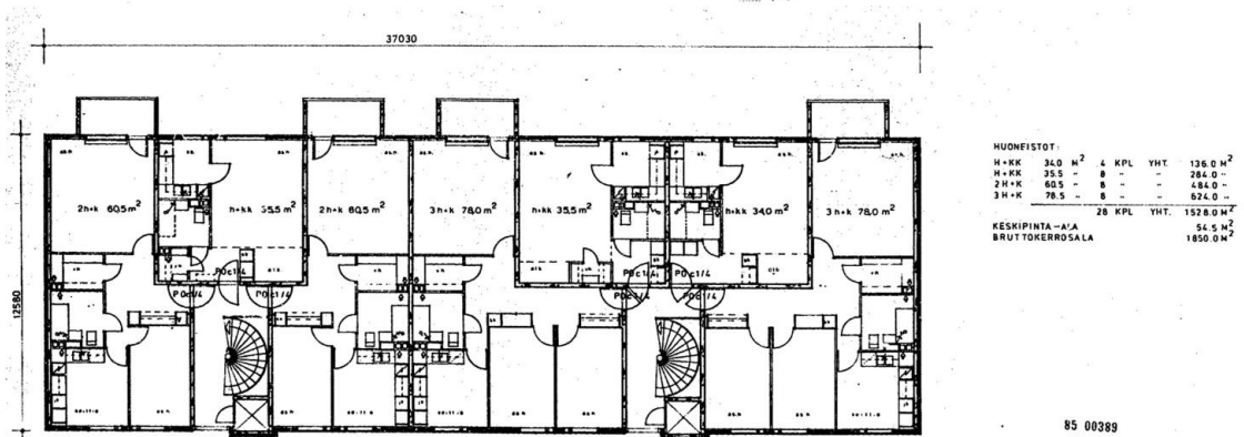
Kuva 13. Tontti 1, talo 1. 1.-4. kerroksen pohjapiirros. Ei mittakaavassa. Kuva RaVa.
