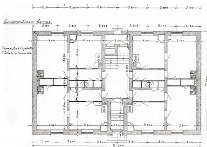
"Lompanlinna", pohjapiirros 1 krs. 13.4.1923
