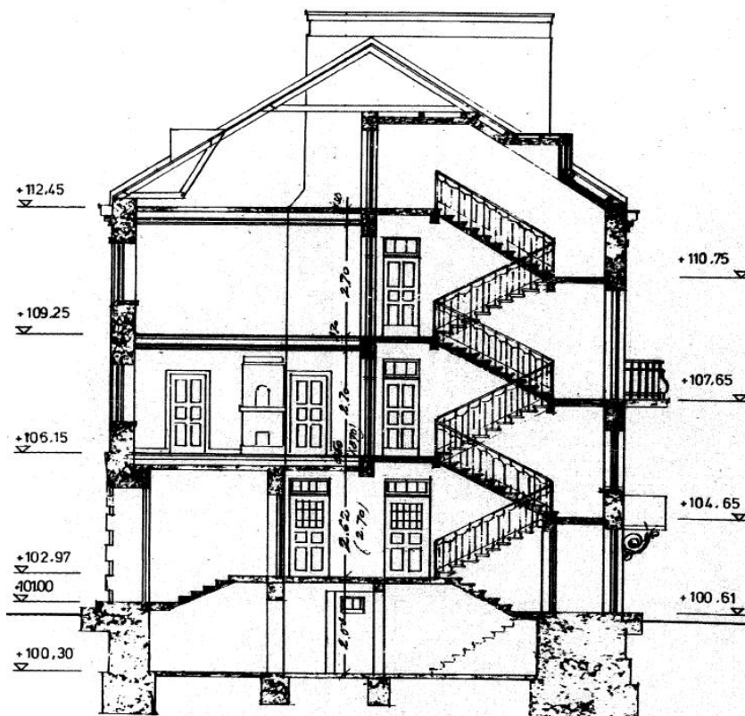
Pajakatu 2, leikkauspiirros 24.6.1986
