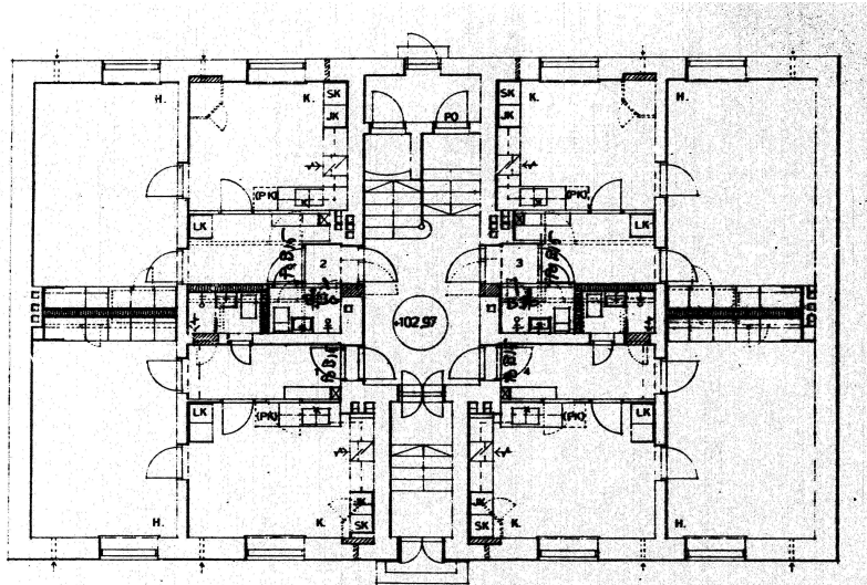
Pajakatu 2, pohjapiirros 1. krs. 24.6.1986
