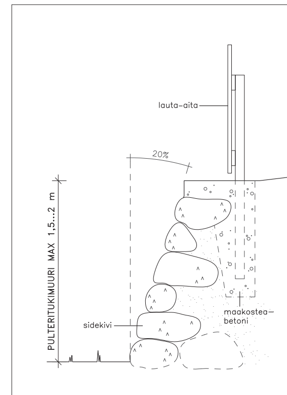
Kylmäladotun pulterimuurin ja siihen yhdistetyn pystysäleaidan periaate.
